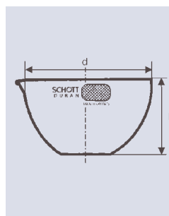
Abdampfschalen mit Ausguss, DIN 12 336
