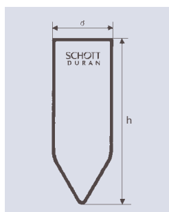
Tubes à centrifuger cylindroconiques en verre DURAN® angle 60°
