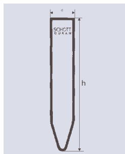
Tube à centrifuger cylindroconique en verre DURAN® angle 30°
