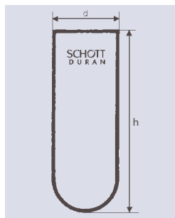
Tubes à centrifuger à fond rond en verre DURAN® DIN 58 970, section 2
